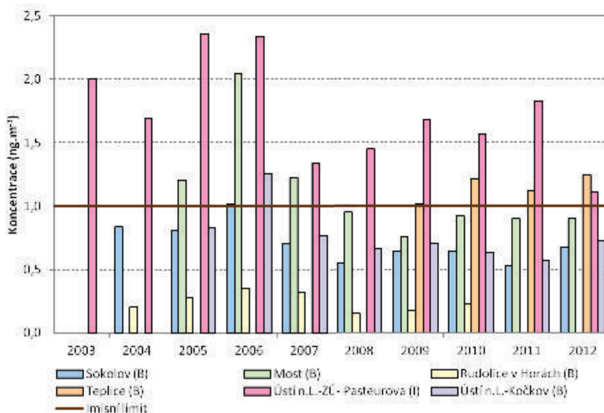
Obrázek 27: Průměrné roční koncentrace benzo(a)pyrenu, zóna CZ04 Severozápad, 2003 – 2012
