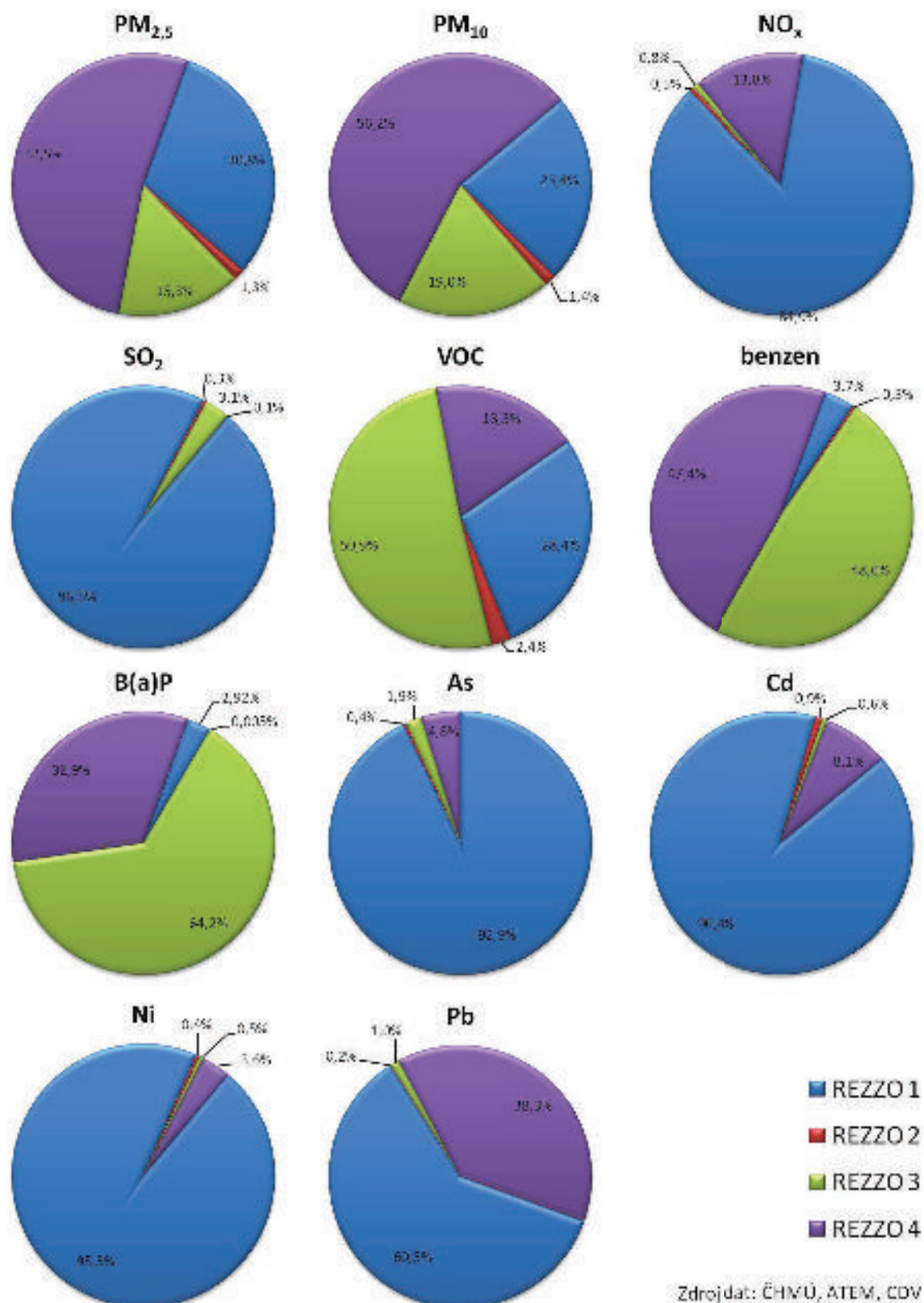
Obrázek 31: Podíl kategorií zdrojů na celkových emisích bilancovaných znečišťujících látek, zóna CZ04 Severozápad, rok 2011 [%]
