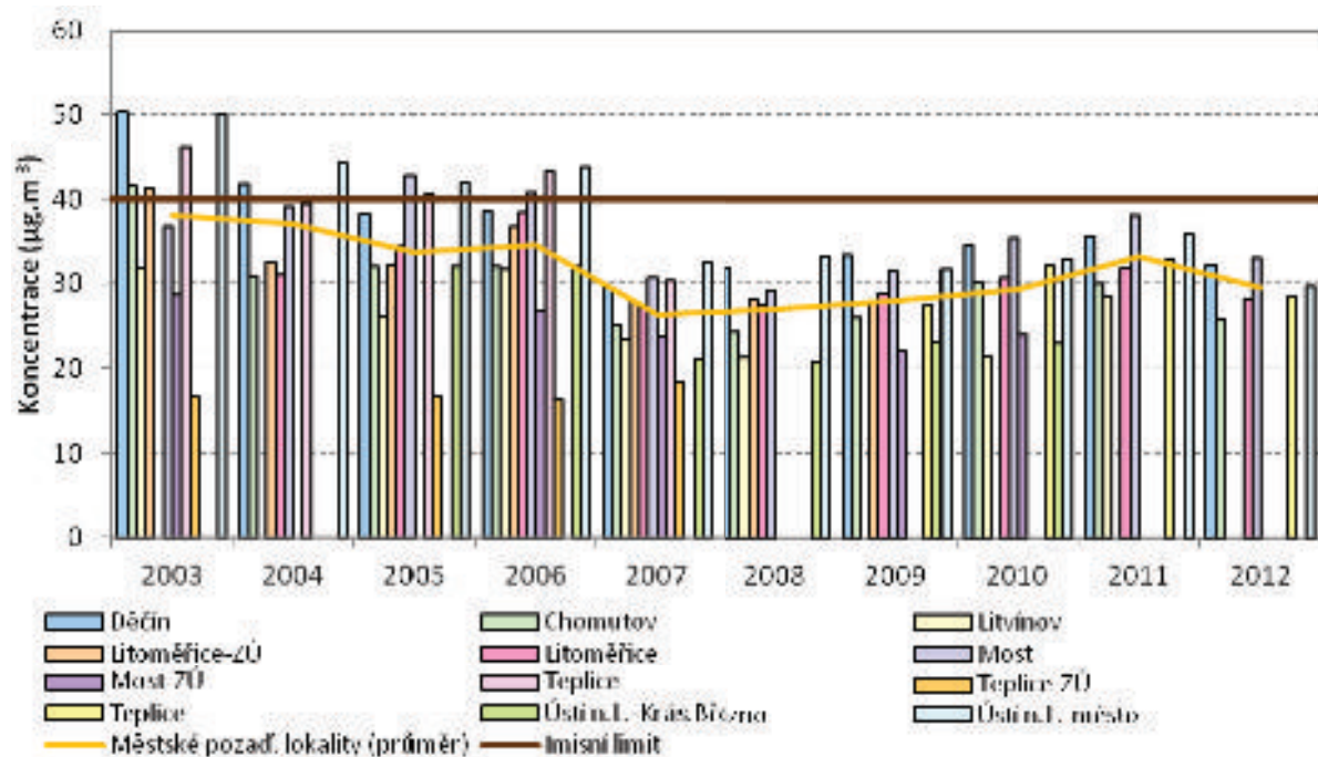
Obrázek 13: Průměrné roční koncentrace PM_{10} na městských pozadíových lokalitách, zóna CZ04 Severozápad, 2003 – 2012
