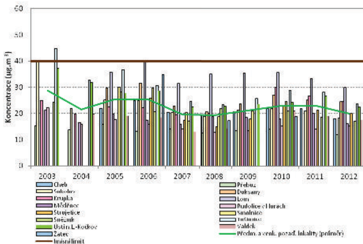
Obrázek 14: Průměrné roční koncentrace PM_{10} na předměstských a venkovských pozadíových lokalitách, zóna CZ04 Severozápad, 2003 – 2012
